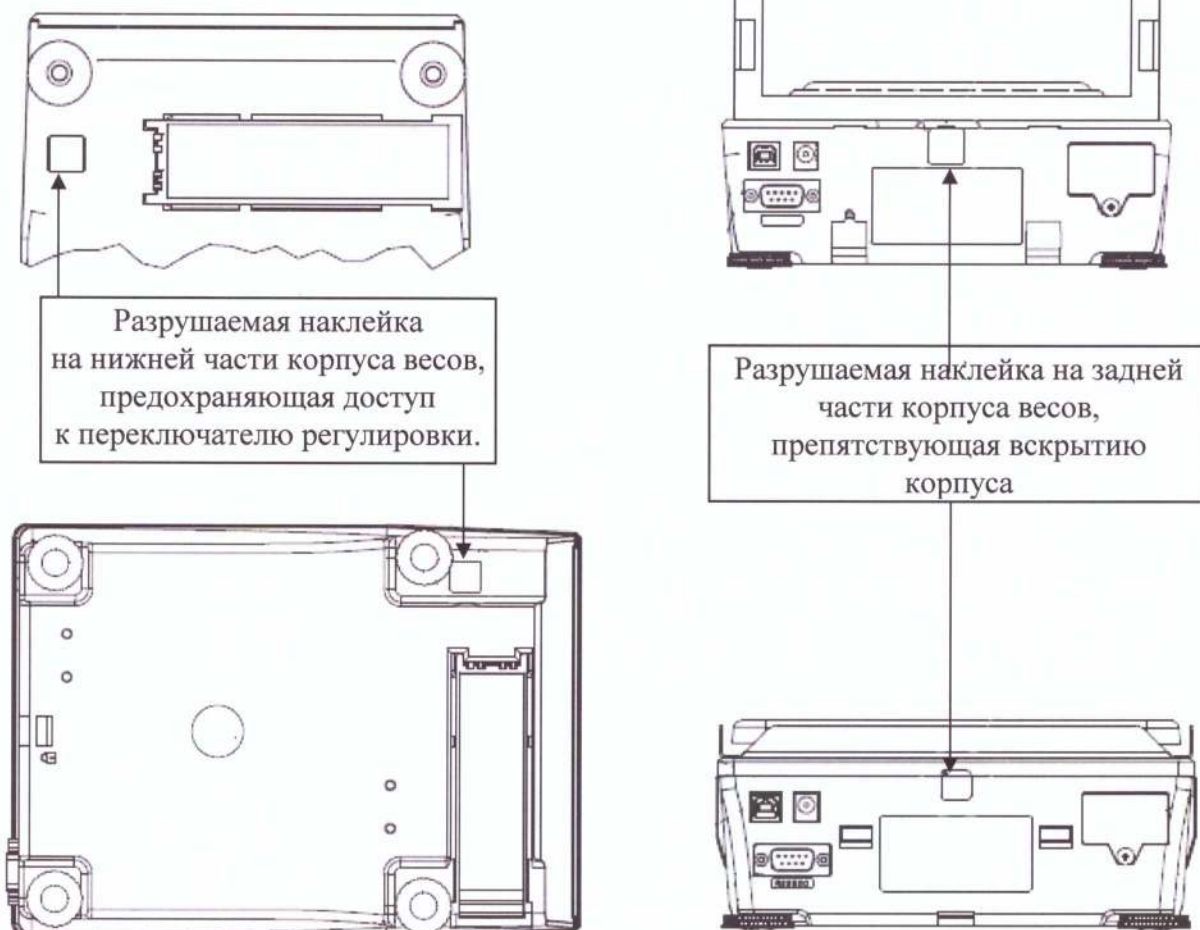
Рисунок 2 - Схема пломбировки весов от несанкционированного доступа
